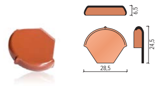
trójkąt początkowy nr 11
