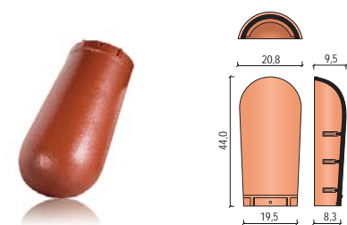
gąsior początkowy grzbietu nr 20
