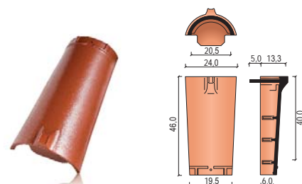
gąsior początkowy kalenicy nr 20
