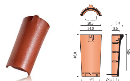
gąsior końcowy kalenicy nr 20
